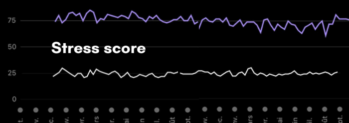
Slaap score
